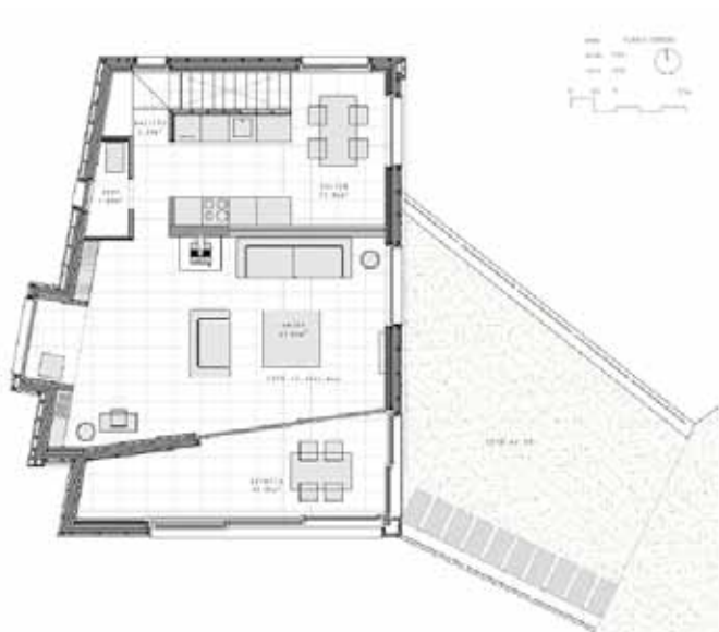
Planta primera
